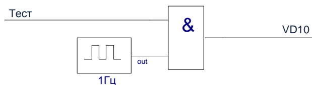
Рисунок 1.2.25– Схема формирования сигнала «Тест»
