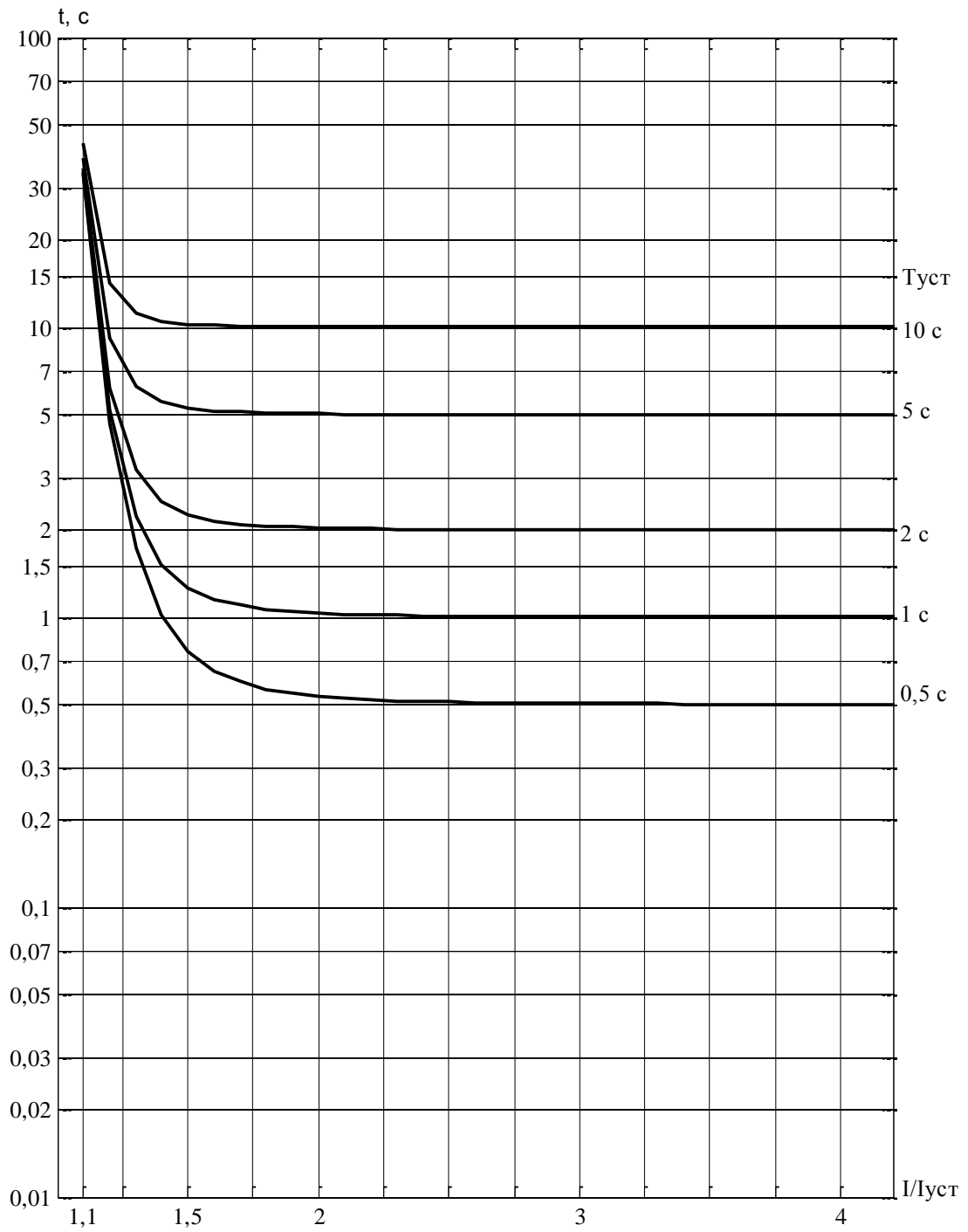
Рисунок Е.6 – Характеристика типа РТВ-I
