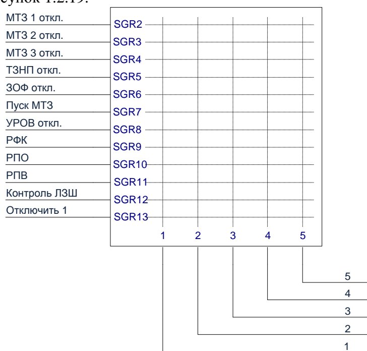
Рисунок 1.2.19 – Логическая схема формирования выходных дискретных сигналов
