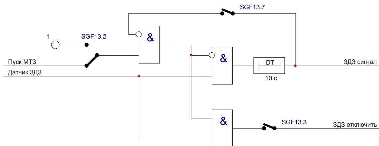
Рисунок 1.2.9 – Логическая схема дуговой защиты
