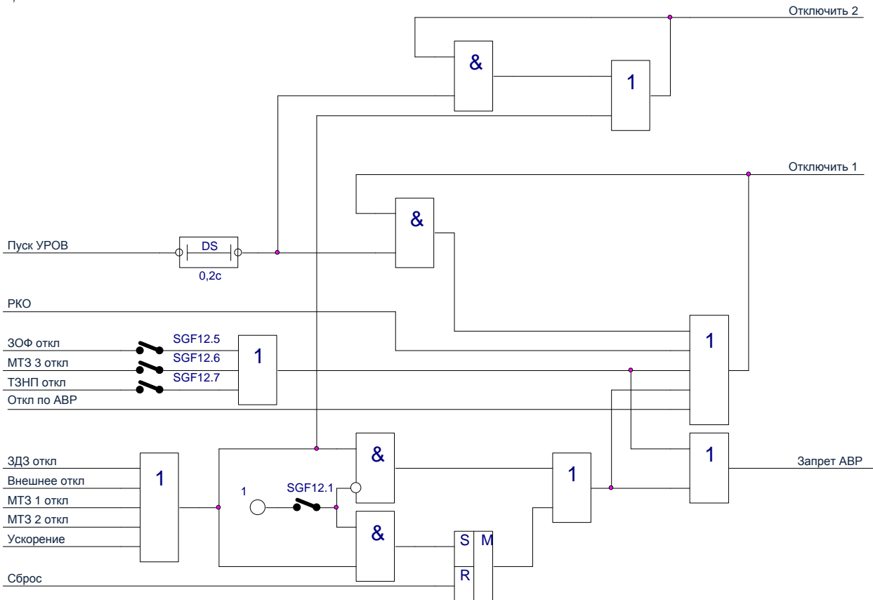
Рисунок 1.2.14 – Логическая схема цепей отключения
