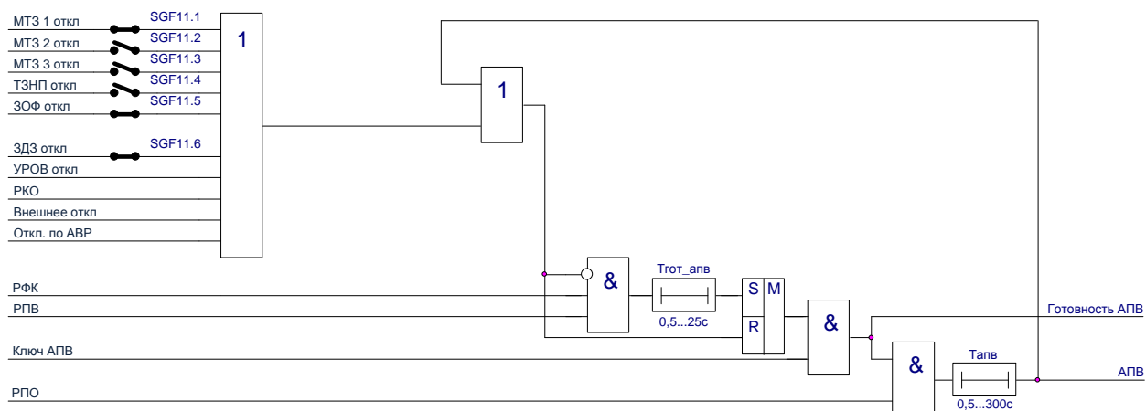
Рисунок 1.2.11 – Логическая схема АПВ
