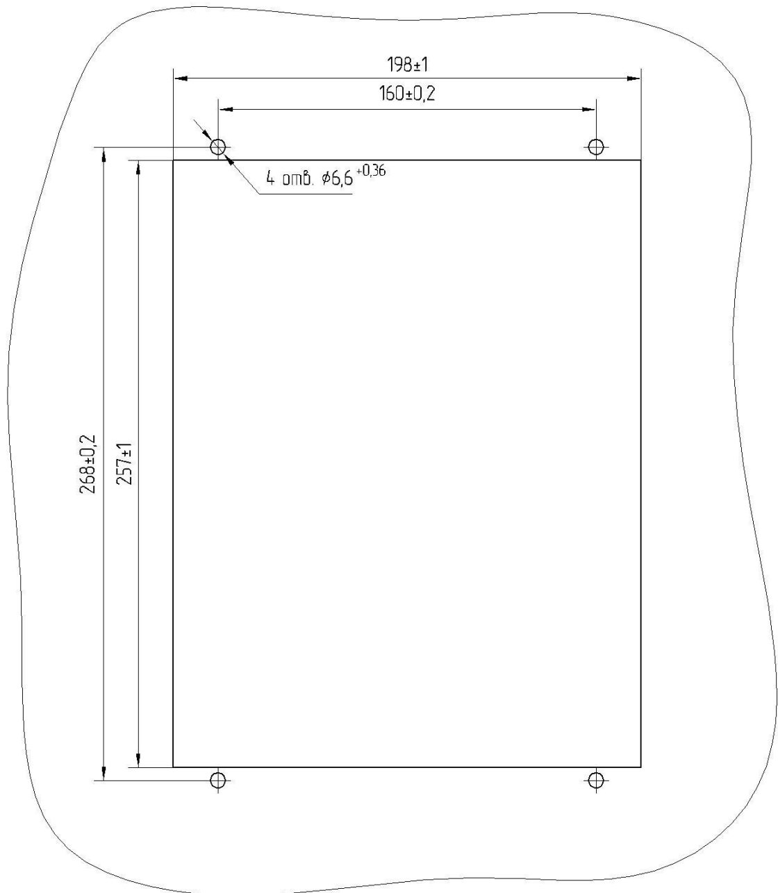
Рисунок А.2 – Отверстие для монтажа TOP 120
