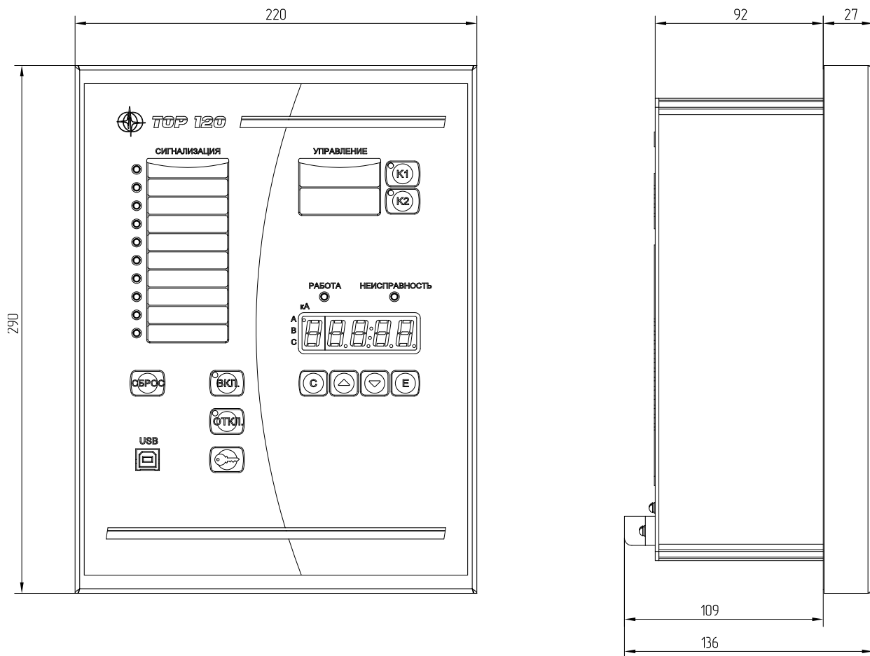
Рисунок А.1 – Габаритные размеры TOP 120
