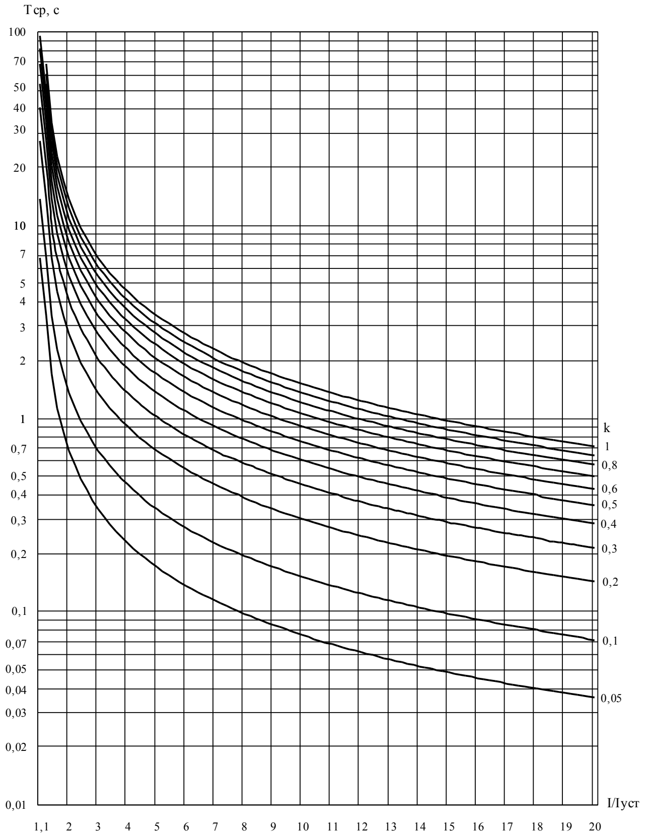
Рисунок Е.2 – Сильно инверсная характеристика
