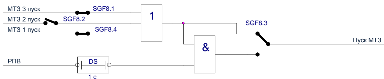
Рисунок 1.2.4 – Логическая схема ЛЗШ
