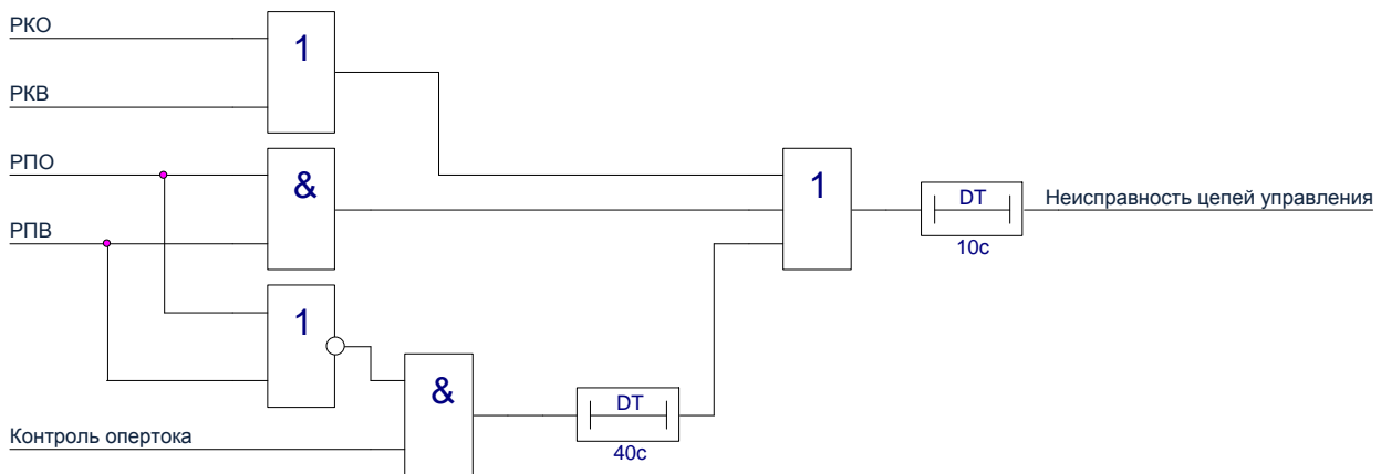
Рисунок 1.2.16 – Логическая схема функционального контроля
