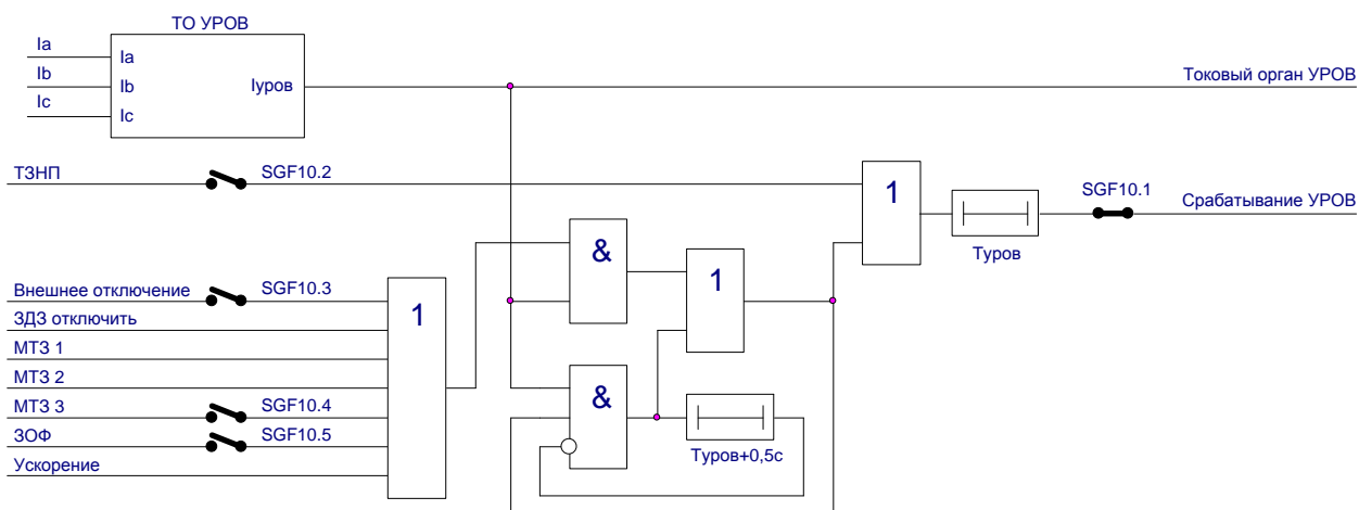
Рисунок 1.2.10 – Обозначение функции УРОВ
