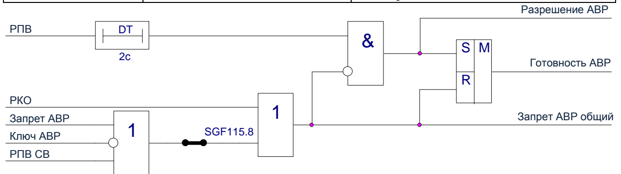
Рисунок 1.2.12 – Схема цепи запрета АВР
