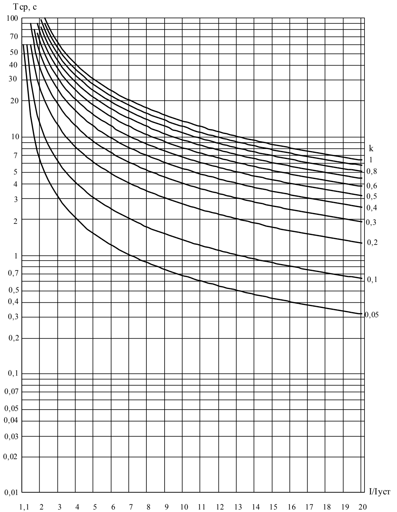
Рисунок Е.4 – Длительно инверсная характеристика
