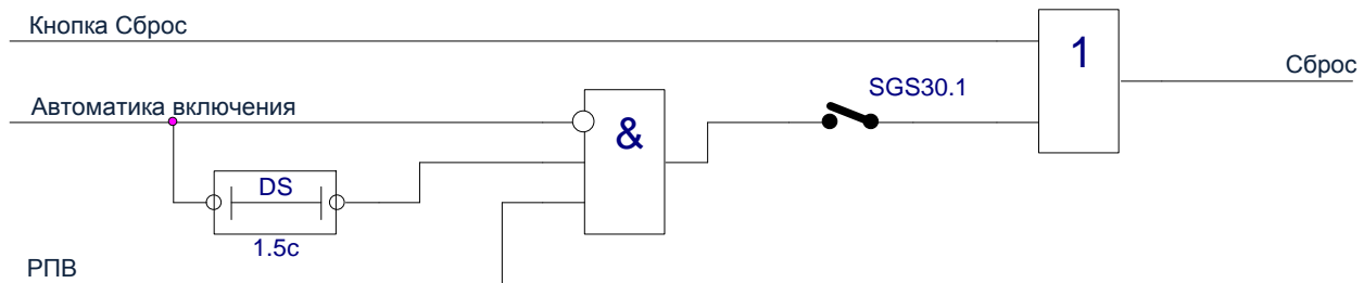
Рисунок 1.2.22 – Логическая схема формирования сигнала «Сброс»
