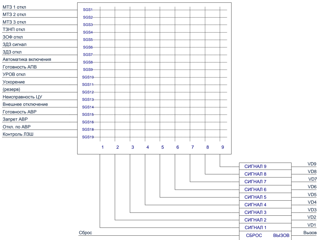
Рисунок 1.2.23 – Логическая схема формирования светодиодной сигнализации
