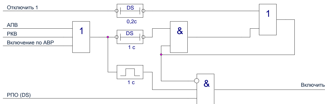
Рисунок 1.2.15 – Логическая схема цепи включения
