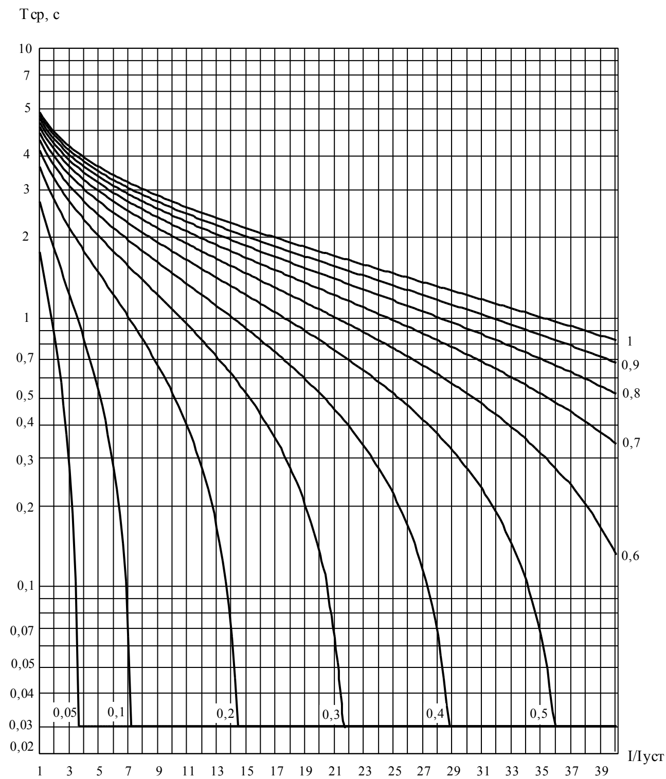
Рисунок Е.5 – Характеристика RXIDG-типа
