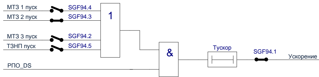
Рисунок 1.2.6 - Логическая схема функции ускорения
