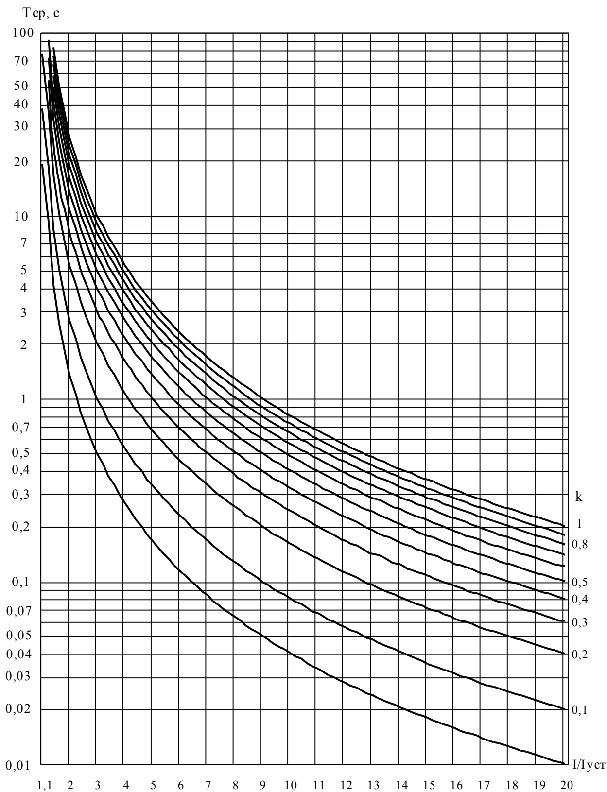
Рисунок Е.1 – Чрезвычайно инверсная характеристика
