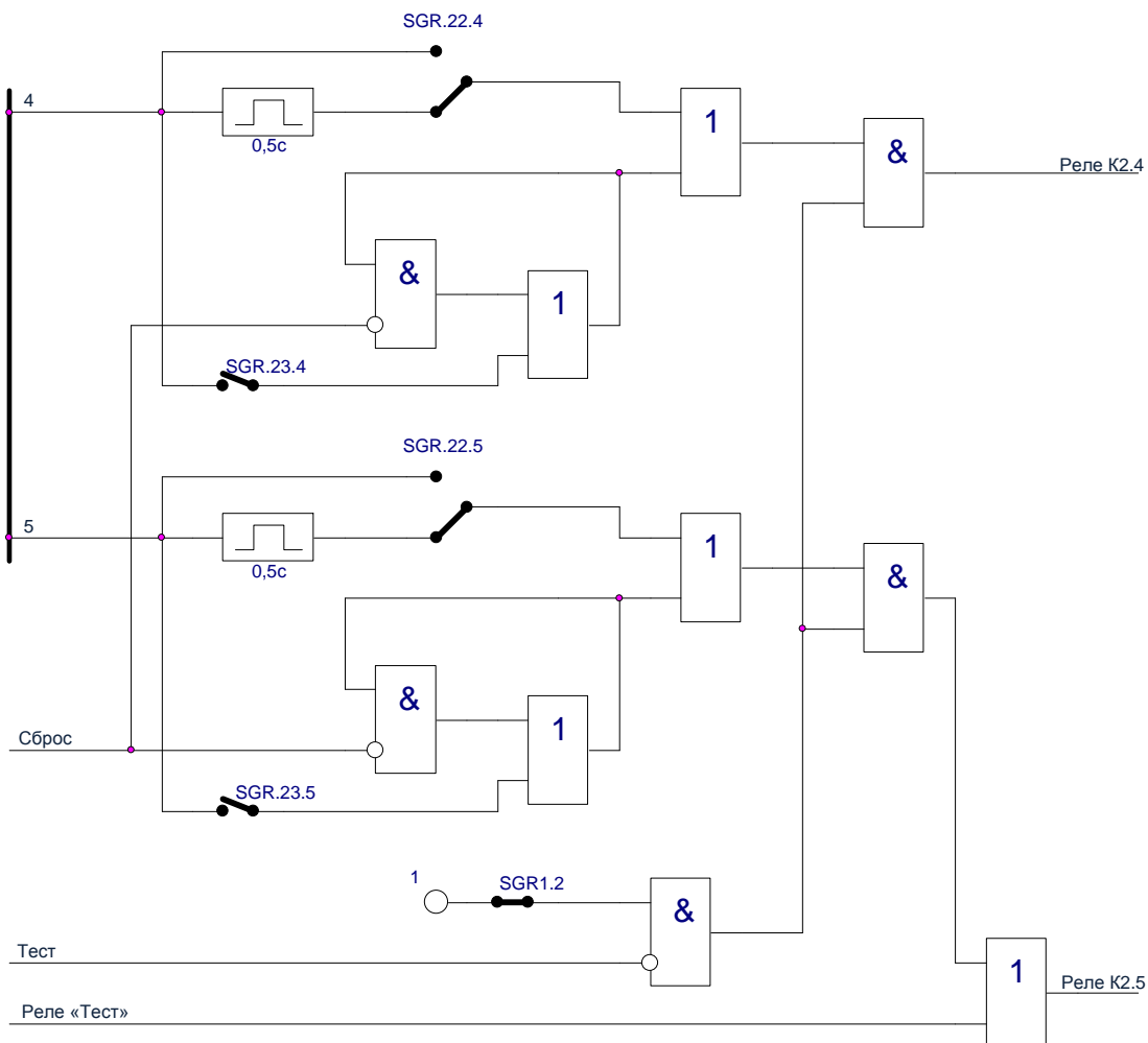
Рисунок 1.2.21 – Логическая схема управления назначаемыми выходными реле
