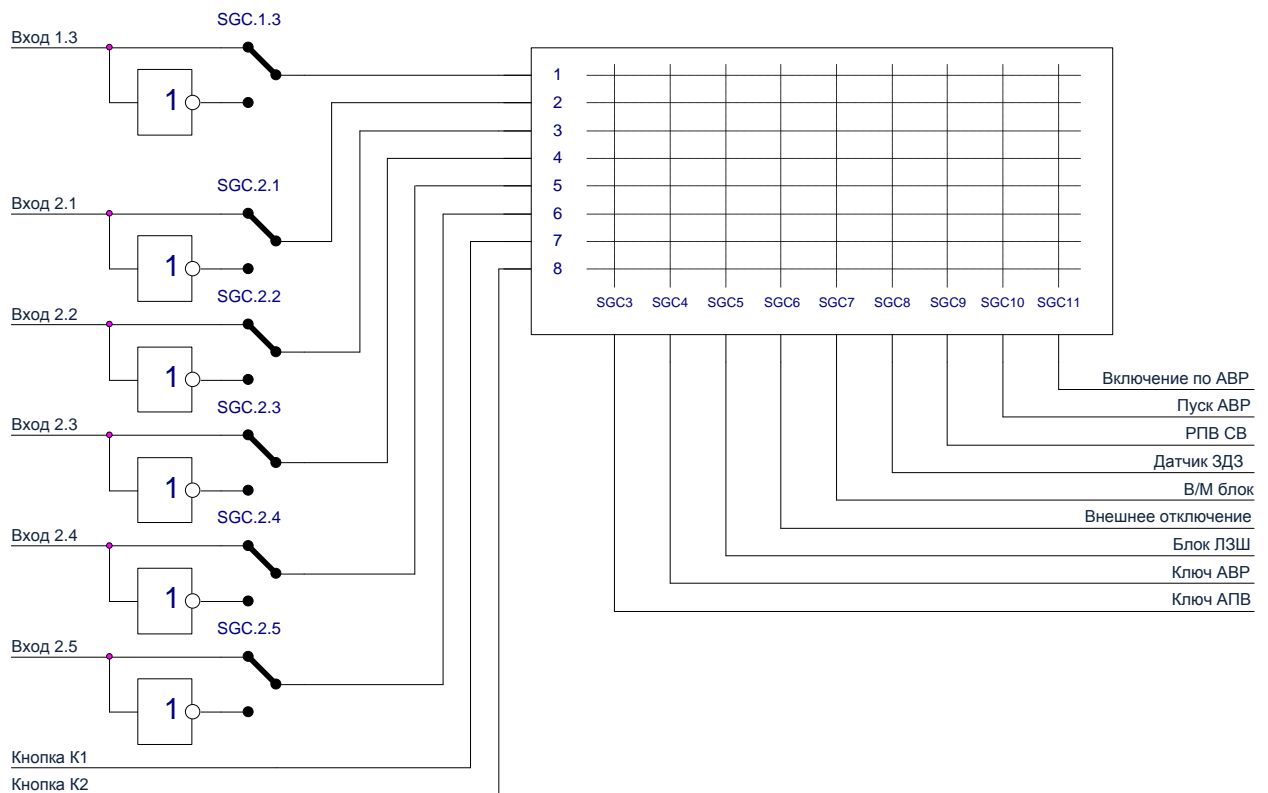
Рисунок 1.2.17 – Логическая схема формирования входных дискретных сигналов
