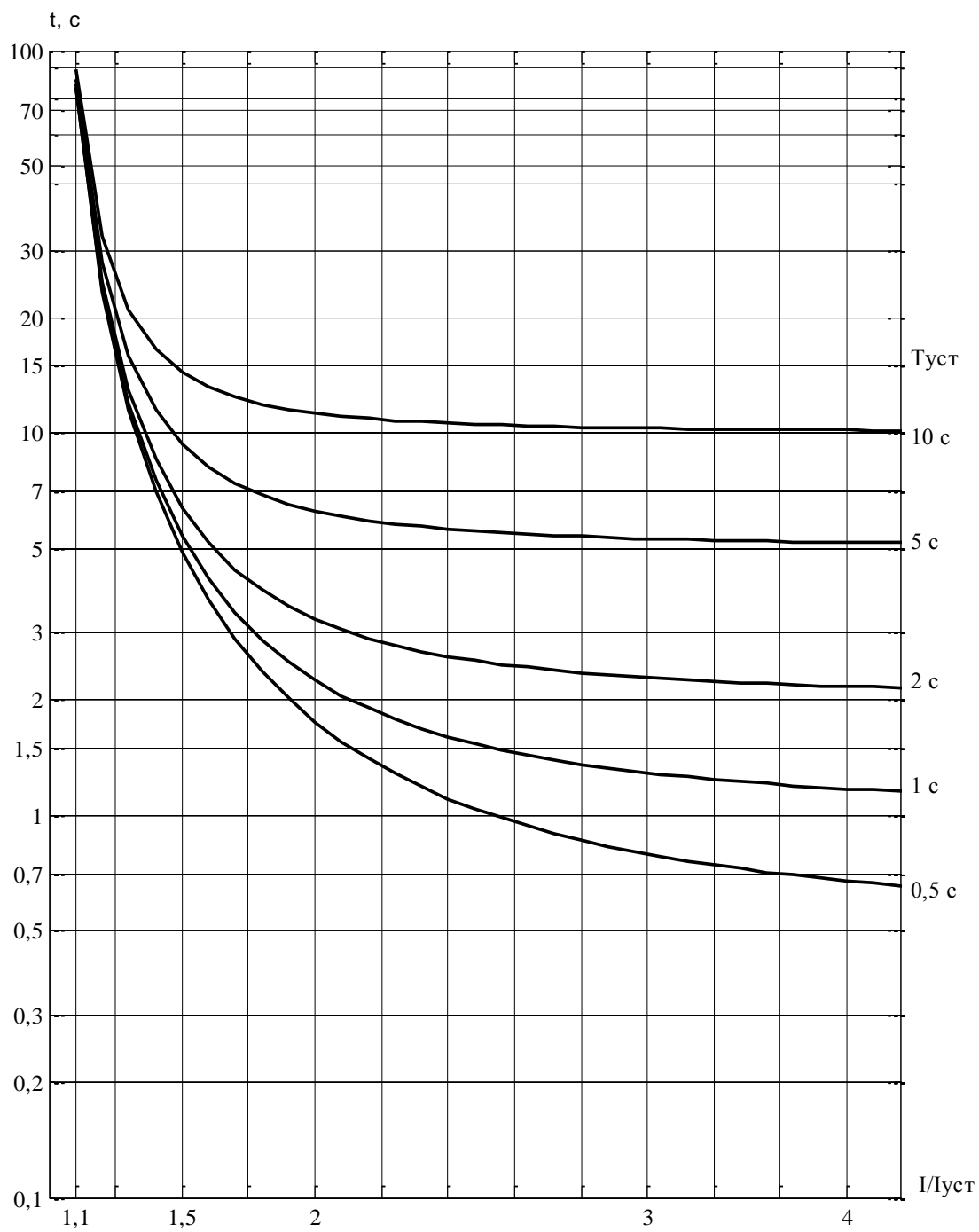
Рисунок Е.7– Характеристика типа РТ-80
