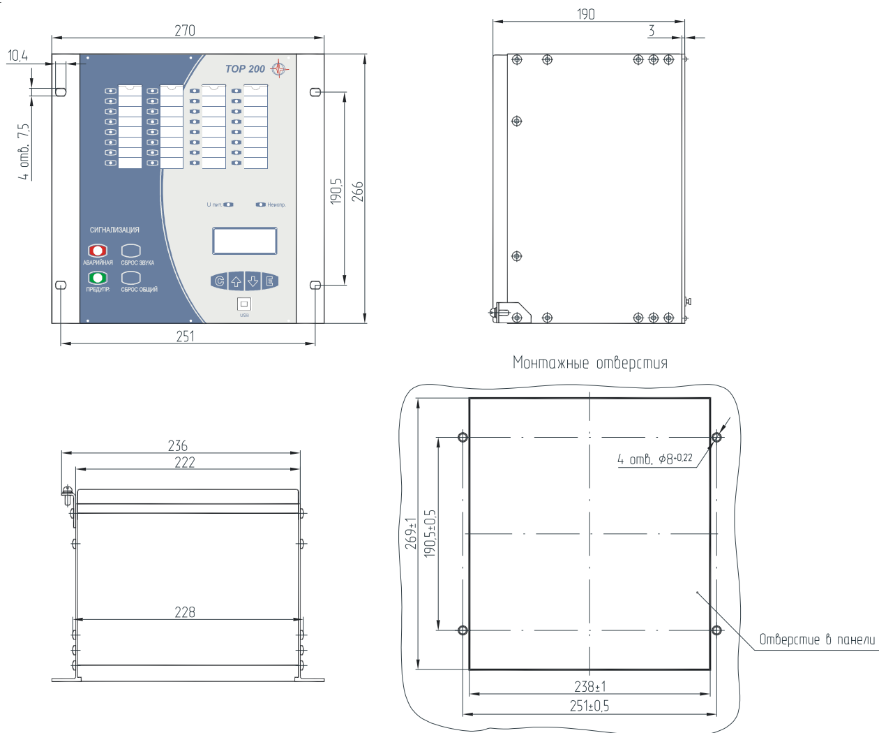
Рисунок В.1 - Габаритные и установочные размеры TOP 200
